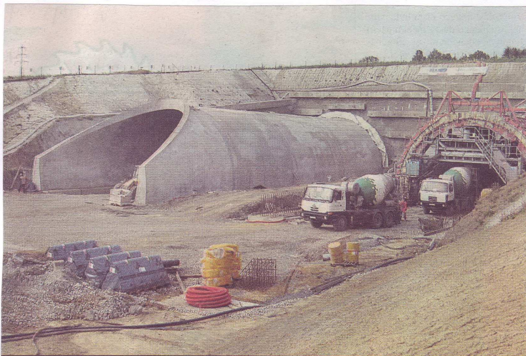
BETON CHRÁNÍ PŘED POŽÁREM. Více než kilometr dlouhý tunel na trase dálnice D47 nedaleko Klimkovic na Ostravsku bude speciálně chráněn proti požáru. Na výstavbu tunelu použili stavaři poprvé v Česku takzvaný protipožární beton s polypropylenovými vlákny, který následky případných požárů snižuje.
